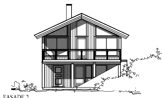
FASADE 2
